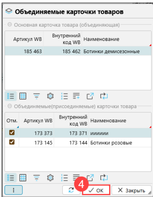
Рис. 14 Подтверждение объединения.
